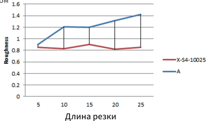
Сравнение изменений тенденций износа инструмента
