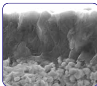
Поперечное сечение инструмента с алмазным покрытием
