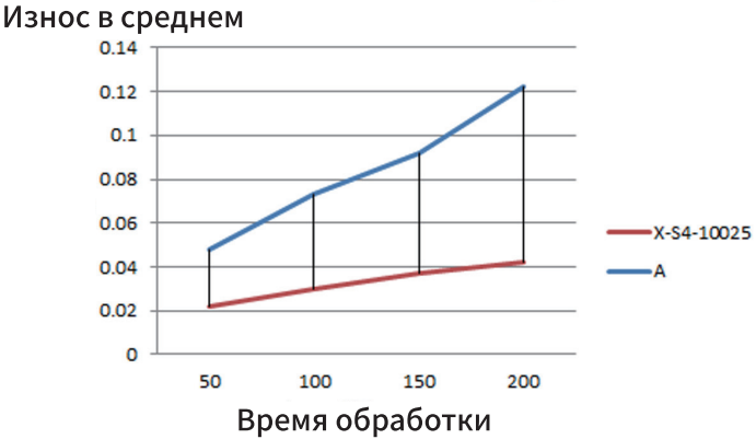
Сравнение изменений тенденций износа инструмента
